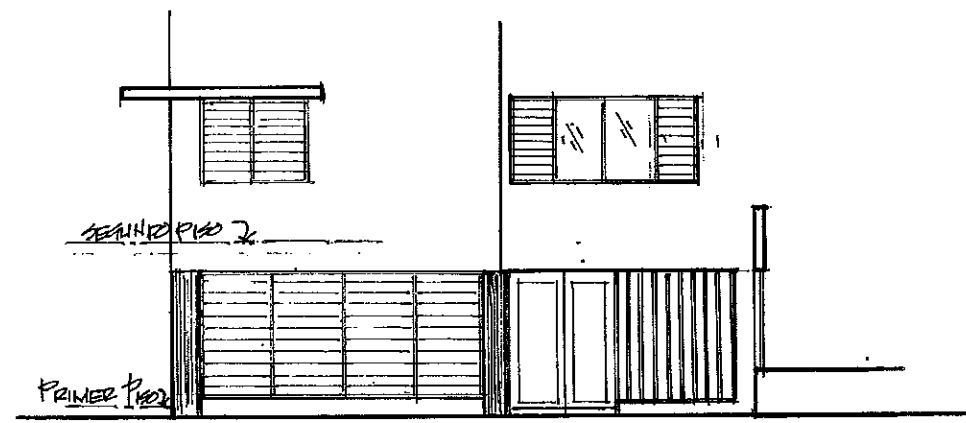
ELEVACION PARCIAL DELANTERA EXISTENTE 1/4" = 1'-0"
