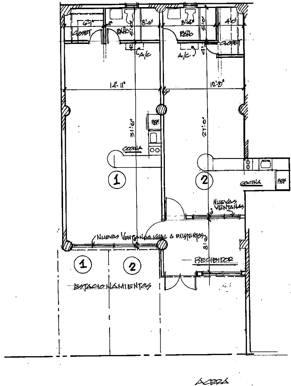
CALLE MARCELA PLANTA PARCIAL PROPUESTA 1/4" = 1'-0"
