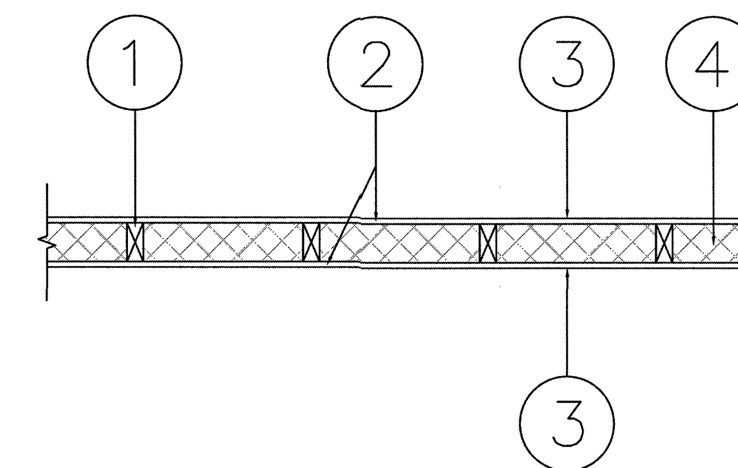
1-HR FIRE WALL (U309) DETAIL N.T.S.
