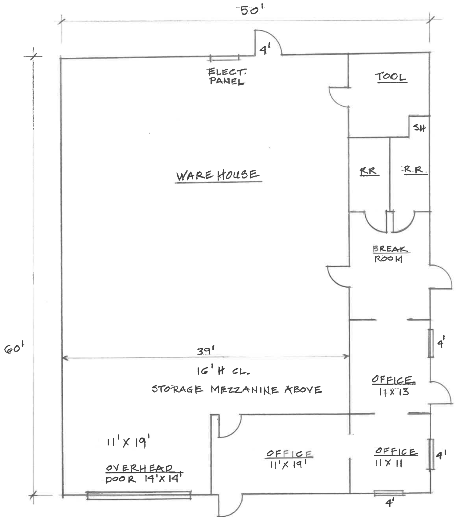
FLOOR PLAN SCALE: 1/8"
